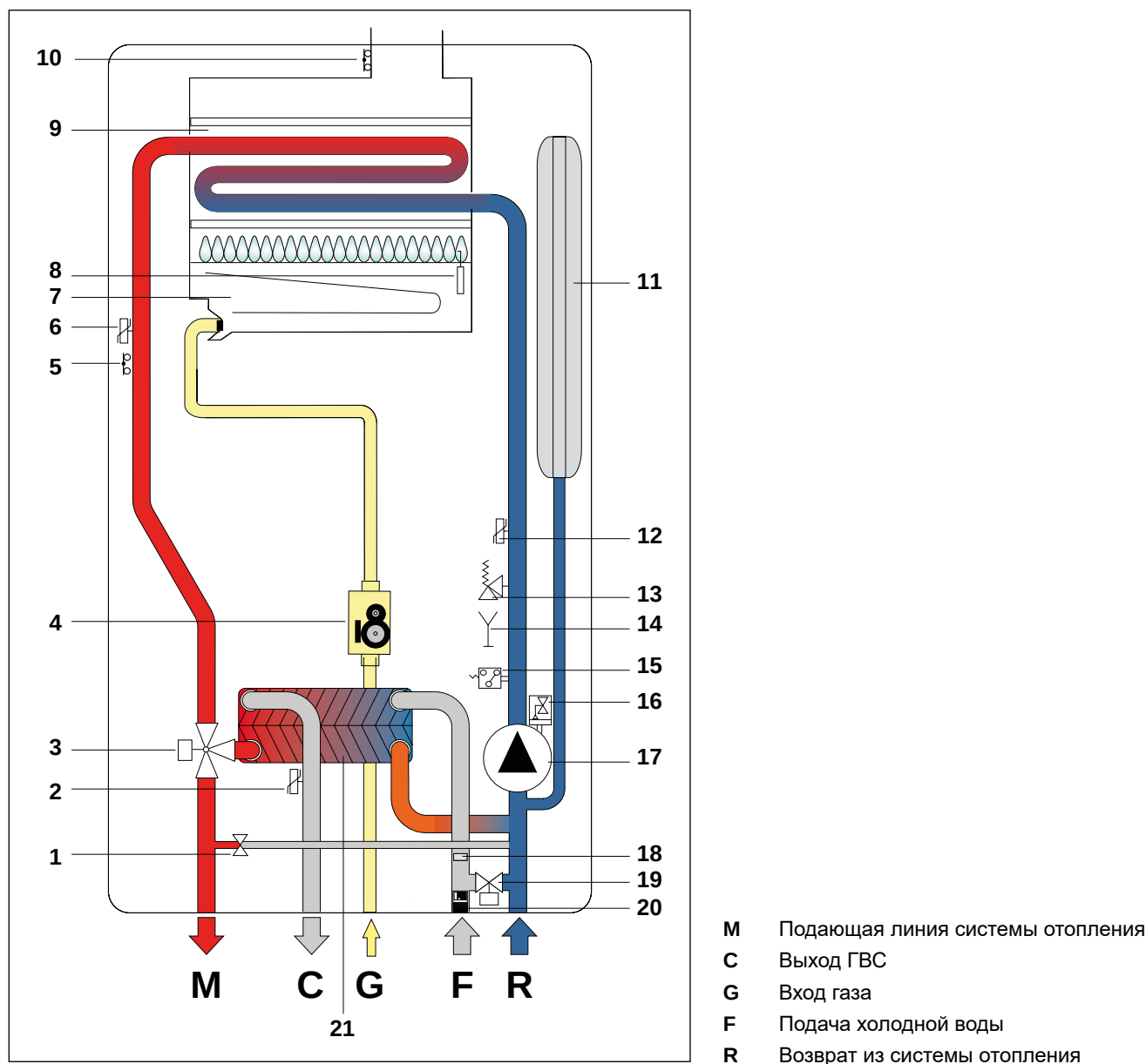
Рис. 6 Гидравлические схемы CTN
